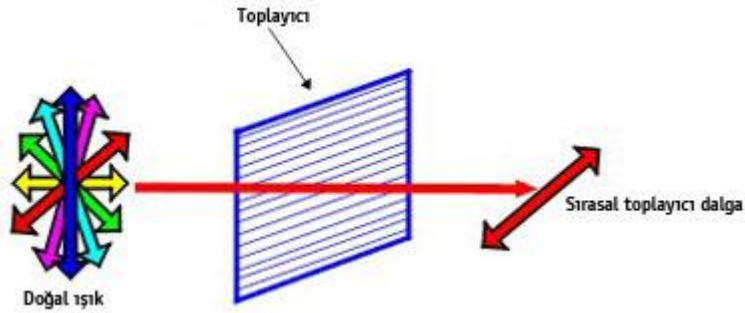
Şekil 3.4: Polarlayıcı yapısı
