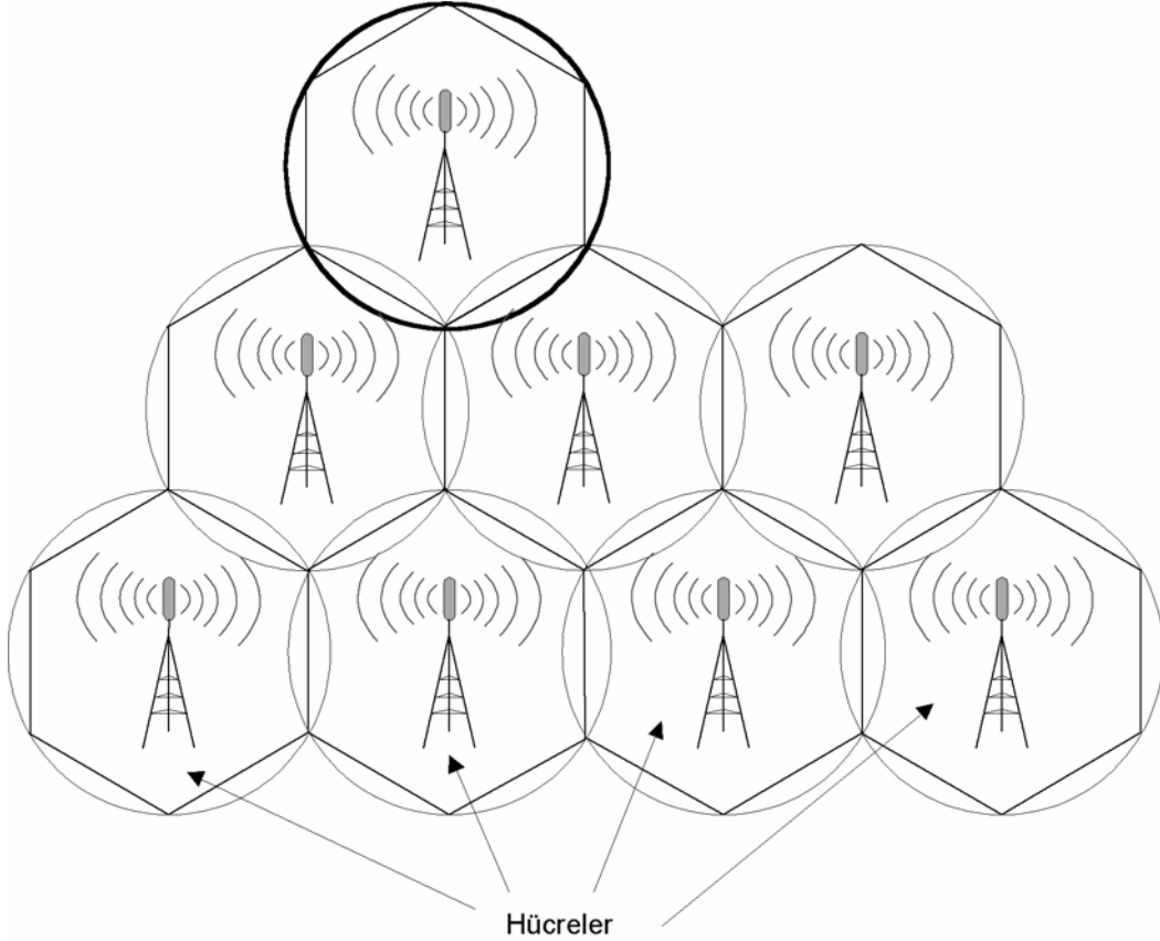
Şekil 5. Hücresel yapı
