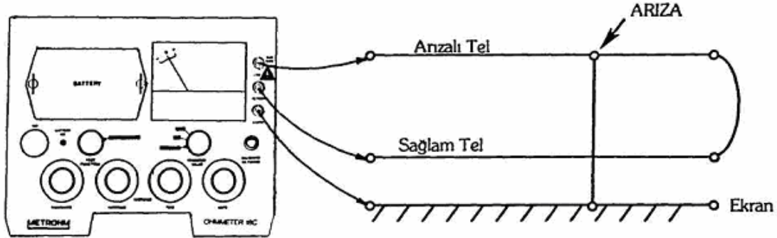
Şekil 2.12: Toprađa temas yerinin bulunması
