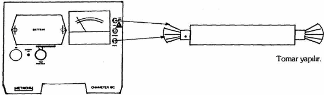
Şekil 2.7: Sağlam iletken kullanarak kopuk arızasının tespiti
