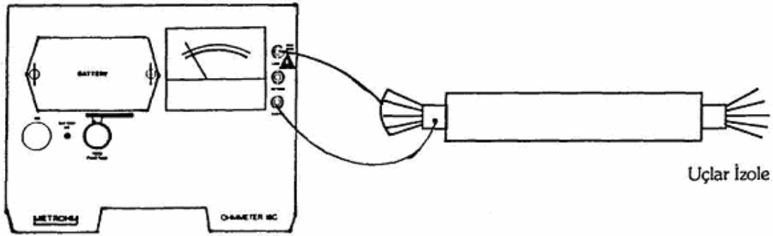
Şekil 2.2: Kablonun toprak arızası ölçümü
