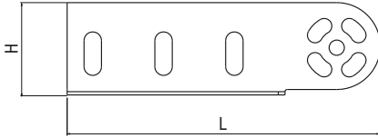
60/75/100 CT-SDE L=160
