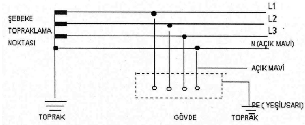
Şekil 1-4 TT Sistemi
