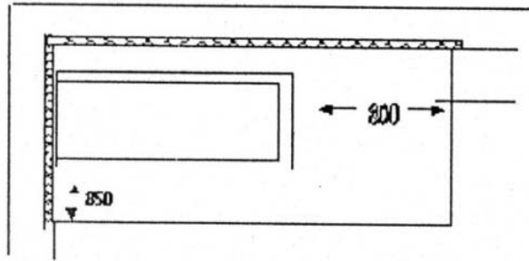
Şekil 21 - Banyoda Koruma Bölgesi
