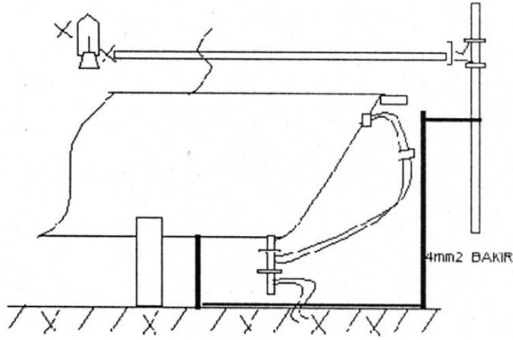
Şekil 22 - Potansiyel Dengelemenin Yapılışı
